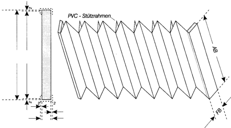
Befestigung der Endflansche von außen
